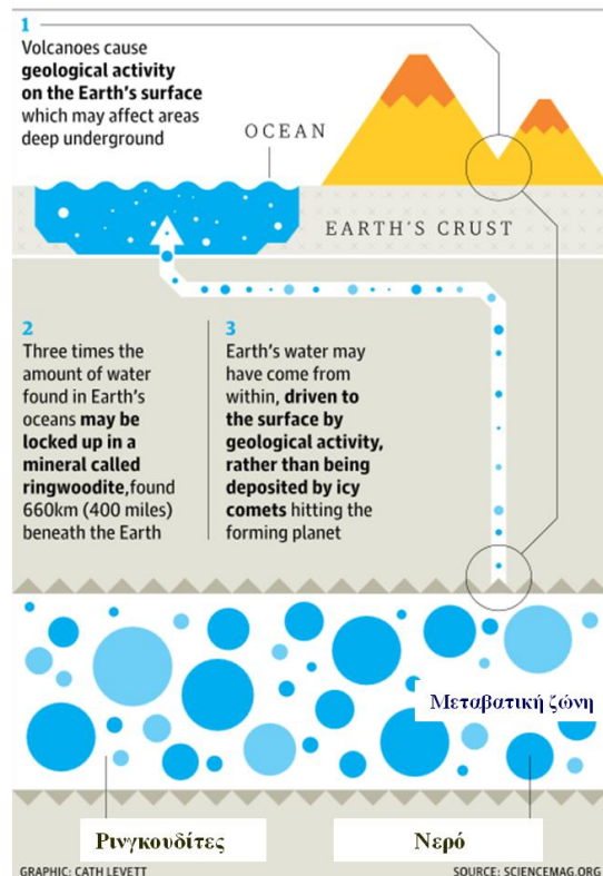
Εικόν 7: Το νερό της Γης παρήχθη (και παράγεται) κυρίως στα έγκατά της.
