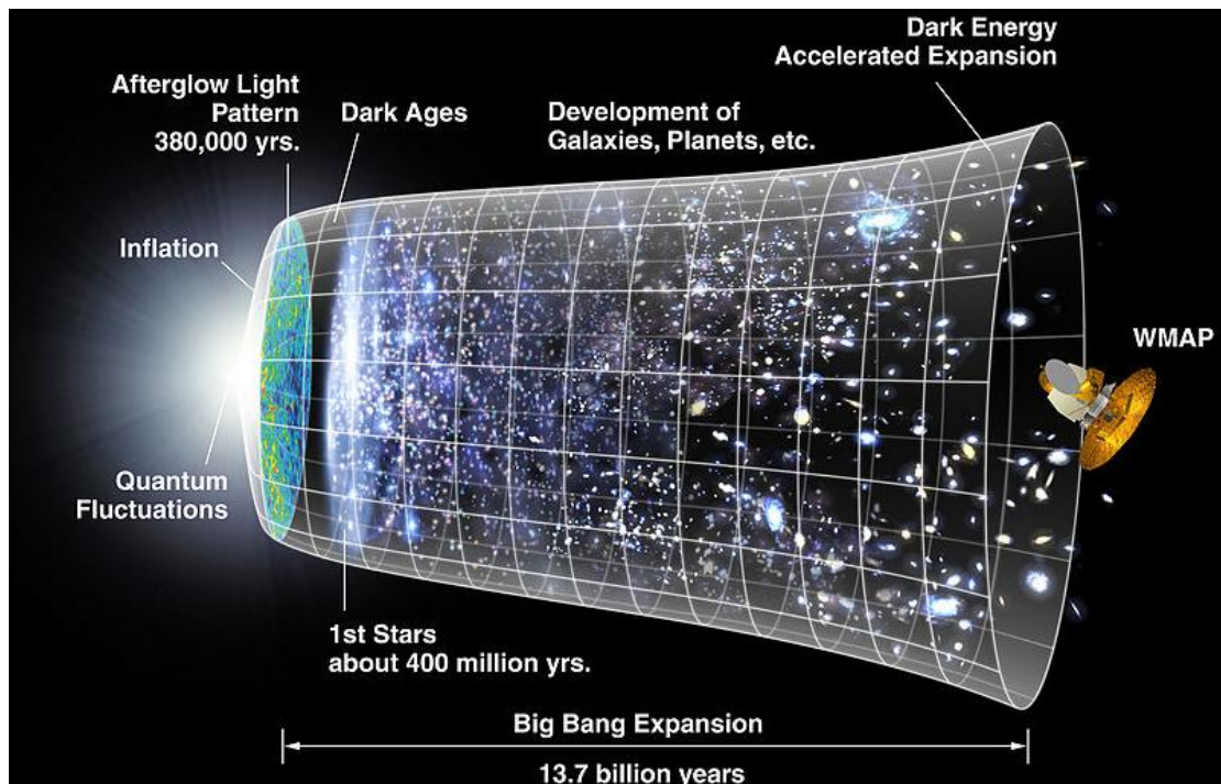
Εικὼν 1: Ἡ διαστολή τοῦ Σύμπαντος μετὰ τὴν Μεγάλῃ Ἐκρηξῇ. Ὁ ὁριζόντιος ἀξὼνας δείχνει τὸν χρόνο. Τὸ Σύμπαν εἰκονίζεται ἀπὸ τὸν κῶδωνα τοῦ σχήματος, ἡ διατομή τοῦ οὗοιου παριστὰ τὸ μέγεθος τοῦ Σύμπαντος τὴν ἀντίστοιχῃ χρονικῇ στιγμῇ. Στὴν ἀρχὴ εἶναι ἓνα "τίποτα", ποῦ εἰκονίζεται ὡς μῖα ἀπειροελάχιστῃ κουκίδα, στὴν ἀρχὴ τοῦ κῶδωνος ἀριστερά. Ἡ ἡμέρα ἡ μῖα ἀρχίζει ὅταν τὸ Σύμπαν φτάνει τὴν ἡλικία τῶν 380000 ἐτῶν· στὴν ἡλικία αὐτῇ τὸ Σύμπαν παριστὰται ἀπὸ τὸν πρᾶσινωπὸ δίσκο ποῦ τέμνει τὸν κῶδωνα τοῦ σχήματος.
