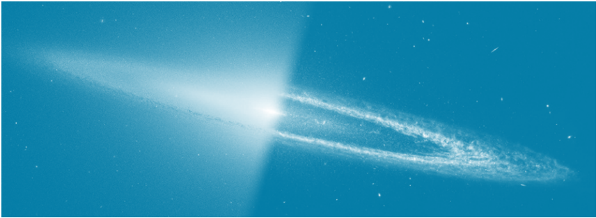
Εικόνα 3: Ο γαλαξίας «Σομπρέρο», όπως φαίνεται με το Webb (δεξιά της εικόνας) και με το Hubble (αριστερά της εικόνας).
