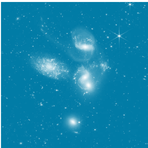
Εικόνα 2: Το «Κουντέτο του Στεφάνου» με τους τέσσερις γαλαξίες.
