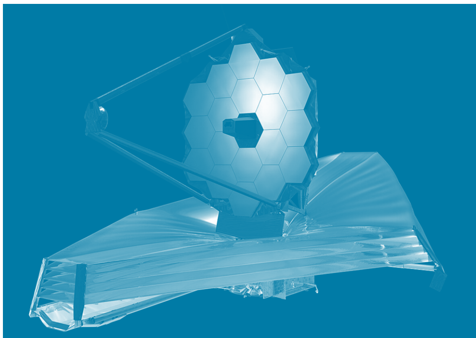
Εικόνα 1: Άποψη του James Webb Space Telescope από το πίσω μέρος, αντίθετο του Ήλιου.
