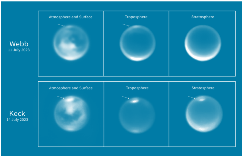
Εικόνα 4: Σύγκριση εικόνων της ατμόσφαιρας, της τροπόσφαιρας και της στρατόσφαιρας του Τιτάν με το Webb και το επίγειο τηλεσκόπιο Keck.
