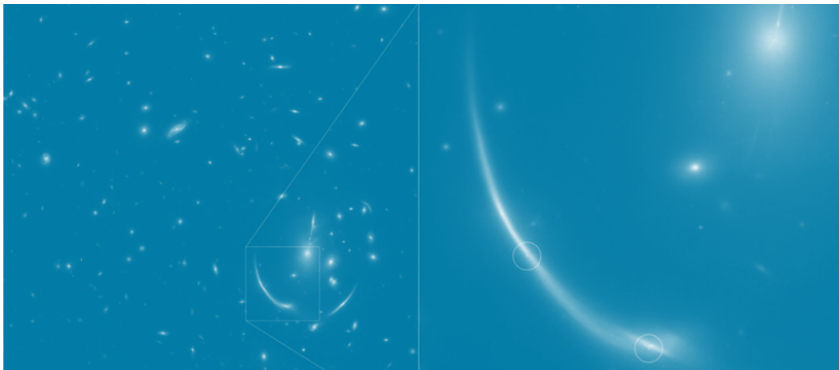
Εικόνα 5: Πολλαπλά απεικονισμένοι σουπερνόβα σε ένα μακρινό γαλαξία, που ονομάζεται, MRG-M0138.
