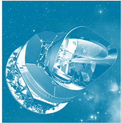
Το διαστημικό τηλεσκόπιο «Planck».
