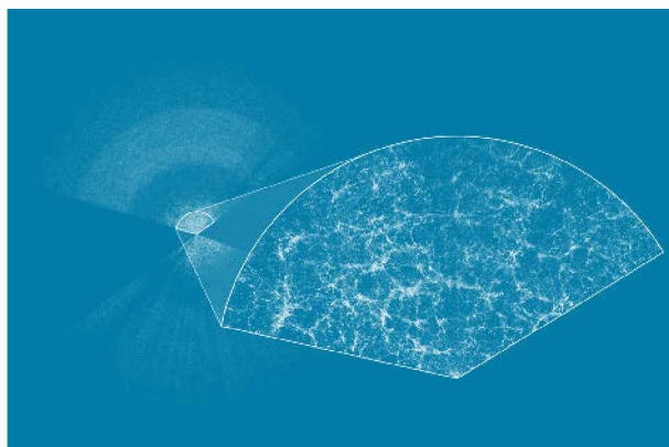
Τμήμα ενός τρισδιάστατου χάρτη μακρινών γαλαξιών του "Sloan". Κάθε κουκίδα αντιπροσωπεύει ένα γαλαξία.
