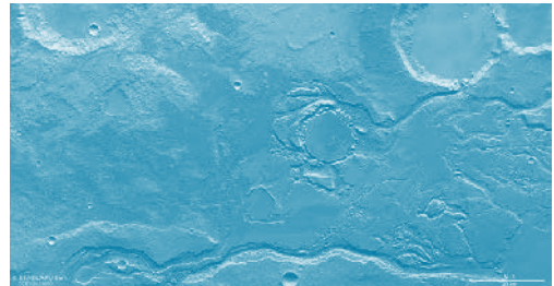
Νεροσυρμές (:) στην επιφάνεια του Άρη
