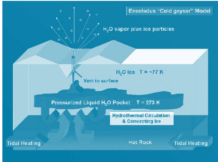
Σχηματική παράσταση πίδακα νερού στον Έγκελαδο, δορυφόρο του Κρόνου
