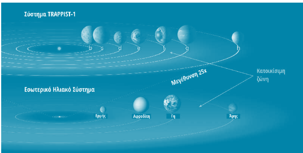
Σχῆμα 5. Οἱ κατοικήσιμες ζώνες γύρω ἀπὸ τὸν TRAPPIST-1 καὶ γύρω ἀπὸ τὸν ἥλιο.
