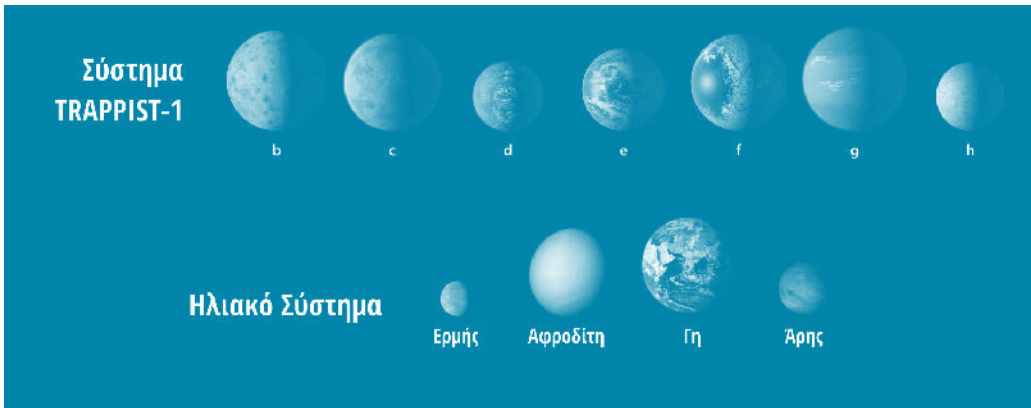
Σχῆμα 4. Οἱ πλανῆτες τοῦ TRAPPIST-1 συγκρινόμενοι με τοὺς ἐσωτερικοὺς πλανῆτες τοῦ ἡλιακοῦ μας συστήματος.
