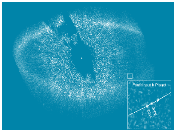
Σχῆμα 3. Ἡ πρώτη ἄμεση παρατήρηση πλανήτη μὲσα σὲ ἕνα νέφος ποὺ περιβάλλει τὸν άστέρα Fomalhaut. Ἡ θέση τοῦ πλανήτη ἀλλάζει ἀπὸ τὸ 2004 στὸ 2006.
