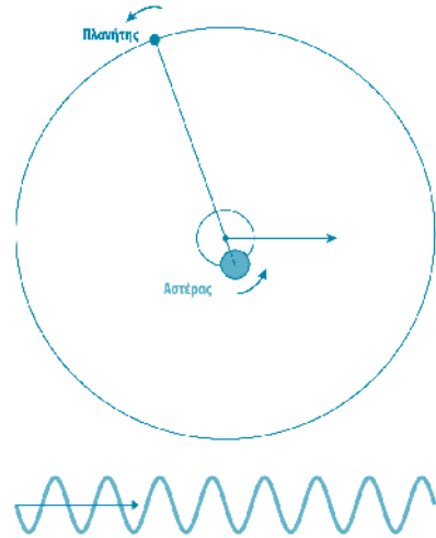
Σχῆμα 1. Ὁ ἀστέρης καὶ ὁ πλανῆτης του περιστρέφονται γύρω ἀπὸ τὸ κοινὸ κέντρο μάζης, τὸ ὁποῖον ἔχει μιὰ εὐθύγραμμη κίνηση. Ἐπομένως, ἡ παρατηρούμενη τροχιά τοῦ ἀστέρα εἶναι μιὰ ταλάντωση γύρω ἀπὸ τὴν εὐθύγραμμη τροχιά.
