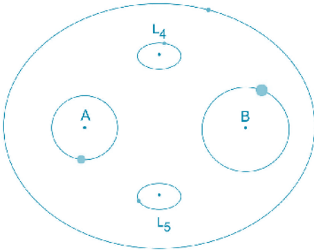
Σχήμα 7. Τροχιές γύρω από ένα ζευγος άστρων A, B.
