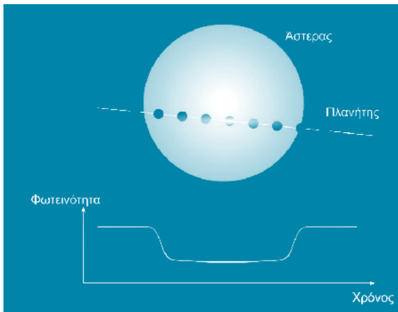
Σχῆμα 2. Όταν ένας πλανήτης διέρχεται μπροστά από τον άστέρα, ἡ λαμπρότης του άστέρα ελαττώνεται.
