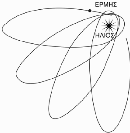
Σχ. 1. Ἡ τροχιά τοῦ Ἑρμοῦ γύρω ἀπὸ τὸν ἥλιο εἶναι περίπου μιὰ ἔλλειψη μὲ συνεχῆ μετάθεσις τοῦ περιηλίου της.
