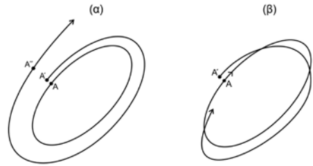
«Σχ. 3. (α) Χαστική τροχιά πλησίον μιας άσταθους περιοδικής τροχιάς. (β) Όργανωμένη τροχιά πλησίον μιας εύσταθους περιοδικής τροχιάς.
