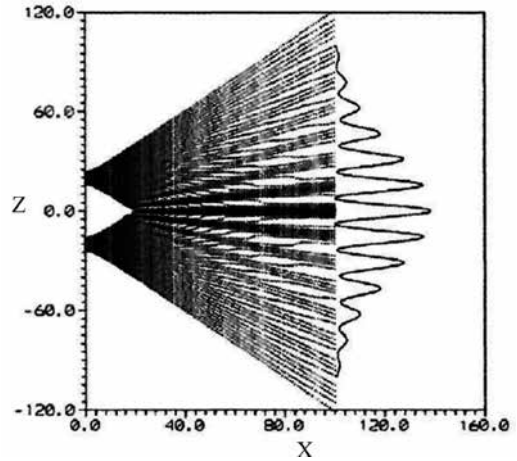
Σχ. 4. Τροχιές σωματιών που διέρχονται από δύο όπες και δημιουργούν κροσσούς συμβολής
