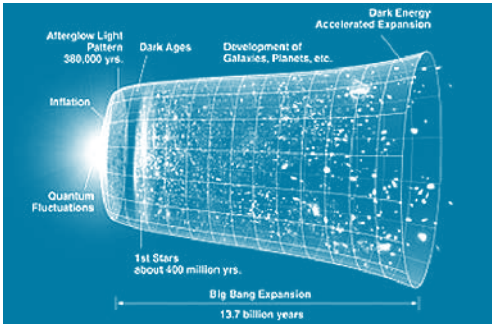
Εικόνα 4: Η ιστορία της διαστολής του Σύμπαντος και της γεννήσεως των αστερών και των γαλαξιών.
