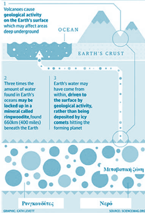
Εικόνα 6: Οί αποθηκευμένοι στη μεταβατική ζώνη ρινγκουδίτες και νερό. Το νερό παριστάται από γαλάζιες φυσαλίδες, και οί ρινγκουδίτες από το λευκό υπόβαθρο. Ο σωλήνας που ένώνει τη μεταβατική ζώνη με τούς ώκεανούς παριστᾶ την ἀπ' εὐθείας γεωλογική μεταφορά τους ἐκεῖ, ἐνῶ οί γραμμές παριστοῦν τὴ μεταφορὰ ρινγκουδιτῶν μέσω ἡφαιστείων.
