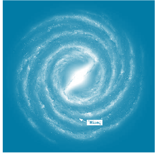
Εἰκόνα 1: Ὁ δικός μας γαλαξίας.
