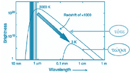
Εἰκόνα 3: Ἡ λαμπρότητα τοῦ ἀρχεγόνου φωτός (κάθετος ἄξονας), ὡς συνάρτηση τοῦ μήκους κύματός του, ὅταν πρωτοέλαμψε καὶ τώρα.
