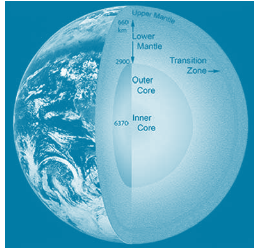
Εικόνα 5: Ὁ ἄνω μανδύας (upper mantle), ἡ μεταβατικὴ ζώνη (transition zone) καὶ ὁ κάτω μανδύας (lower mantle).
