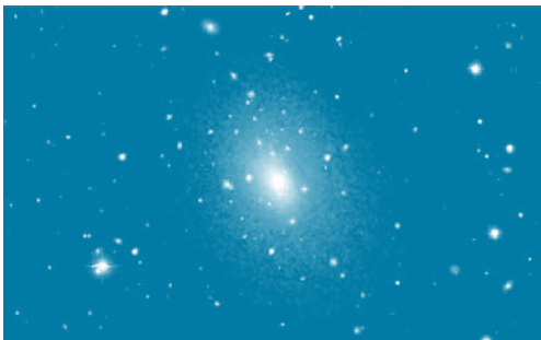
Εικόνα 2: Τὸ σμήνος γαλαξιών Abel 2029.
