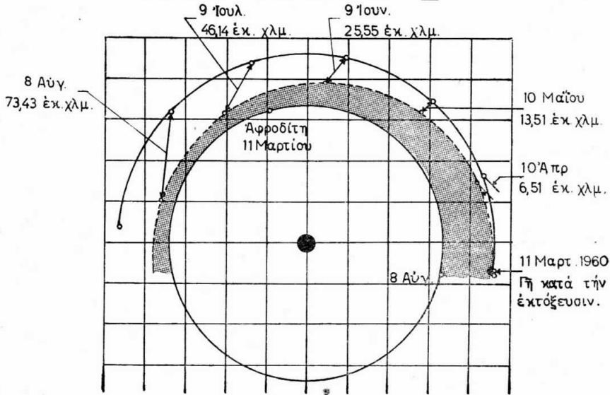
Τροχιά τοῦ Πρωτοπόρου V περὶ τὸν Ἡλιον (ἔστιγμένη γραμμή), τῆς Γῆς (ἐξωτερικὴ καμπύλη) καὶ τῆς Ἀφροδίτης.
