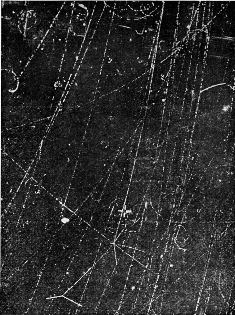
Εικ. 4. Ἐκμηδενισμός άντι—πρωτονίου. Τοῦτο ερχόμενον ἐκ τῶν άνω συναντᾶται με ἕνα πρωτόνιον άνθρακος και δημιουργεῖται ἕνα θραῦσμα ὑπό μορφήν «άστέρου». Κάτω άριστερά ἕνα πρωτόνιον άναπηδᾷ κατά τήν σύγκρουσιν με ἕνα μεσόνιον.
