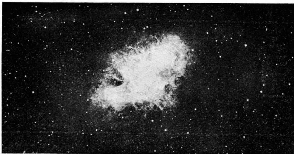
Εἰκ. 5. Ὁ νεφελοειδὴς τοῦ Καρκίνου διὰ τοῦ τηλεσκοπίου τοῦ Ὁρους Οὐτίλων. Πιθανῶς τὸ φῶς τοῦ προέρχεται ἀπὸ σωματῖα δημιουργηθέντα ἀπὸ τὸν ἐκμηδενισμὸν τῆς άντι-ύλης.
