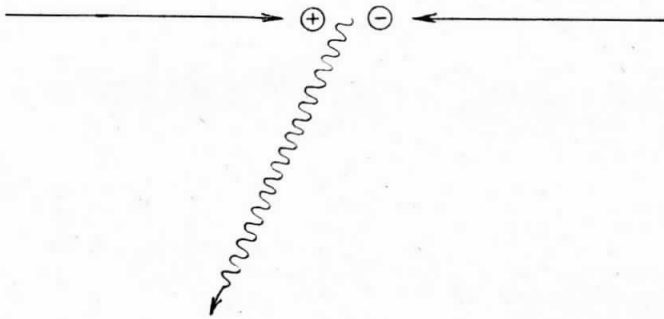
Εἰκ. 3. Σύγκρουσις ἠλεκτρονίου καὶ ἀντι-ἠλεκτρονίου ἐπιφέρει τὸν ἐκμηδενισμόν τῆς μᾶζης καὶ τῶν δύο. Ὅταν αὐτὰ συγκρουσθῶν μέσα εἰς τὸ ἄτομον, ἡ μᾶζα τῶν θά μετατραπῇ εἰς ἓνα φωτόνιον, ἂν δὲ γίνῃ εἰς τὸν ἐλεύθερον ζῶρον θά ἐκπεμφθῶν δύο φωτόνια.
