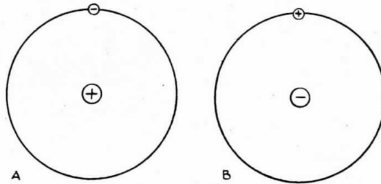
Εἰκ. 2. Ἡ Α παριστᾶ ἄτομον ὑδρογόνου μέ τόν πρωτόνιον εἰς τόν κέντρον και τόν ἠλεκτρόνιον εἰς τήν περιφέρειαν. Ἡ Β παριστᾶ ἄτομον άντι-ὑδρογόνου ἔχον εἰς τόν κέντρον τόν ἀντιπρωτόνιον και εἰς περιφέρειαν τόν άντι - ἠλεκτρόνιον.
