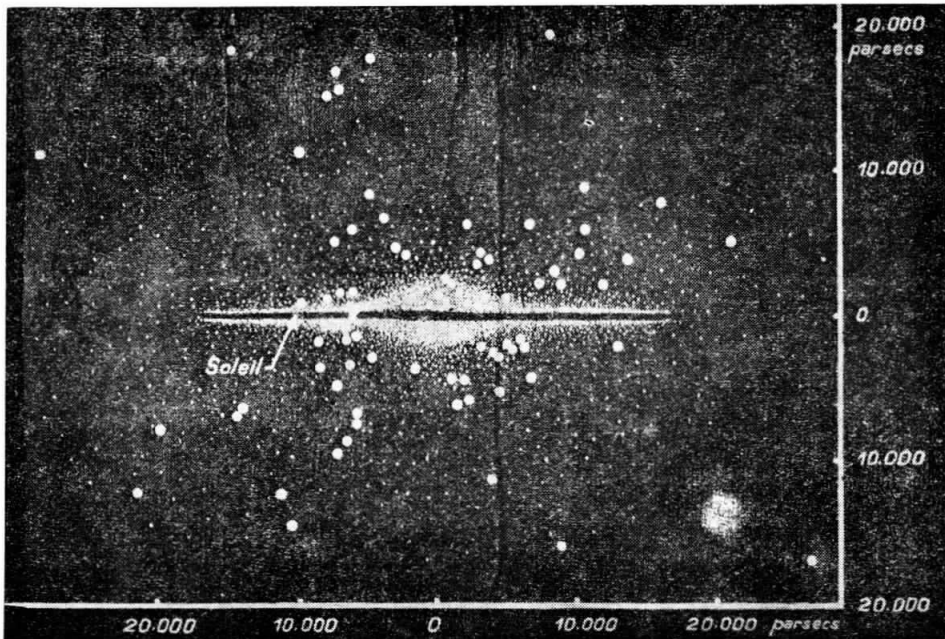
Εἰκ. 5. Σχηματικὴ μορφή τοῦ γαλαξιακοῦ μας συστήματος ὅπως θὰ ἐφαίνετο ἐκ τῶν πλαγίων. Διακρίνεται τὸ κεντρικὸν ἐπίπεδόν του ἐκατέρωθεν τοῦ ὁποίου οἱ ἀστέρες εἶναι πολὺ πλησίον ἀλλήλων. Οἱ ἐγκατεσπαρμένοι μεγάλοι λευκοὶ κύκλοι εἶναι τὰ σφαιρωτὰ σμήνη καὶ οἱ μικροὶ κύκλοι οἱ μεταβλητοὶ ἀστέρες τύπου RR. Lyr. Ἀριστερά, ἄνωθεν τοῦ ἐπιπέδου, διακρίνεται ἡ θέσις τοῦ Ἡλίου μας.
