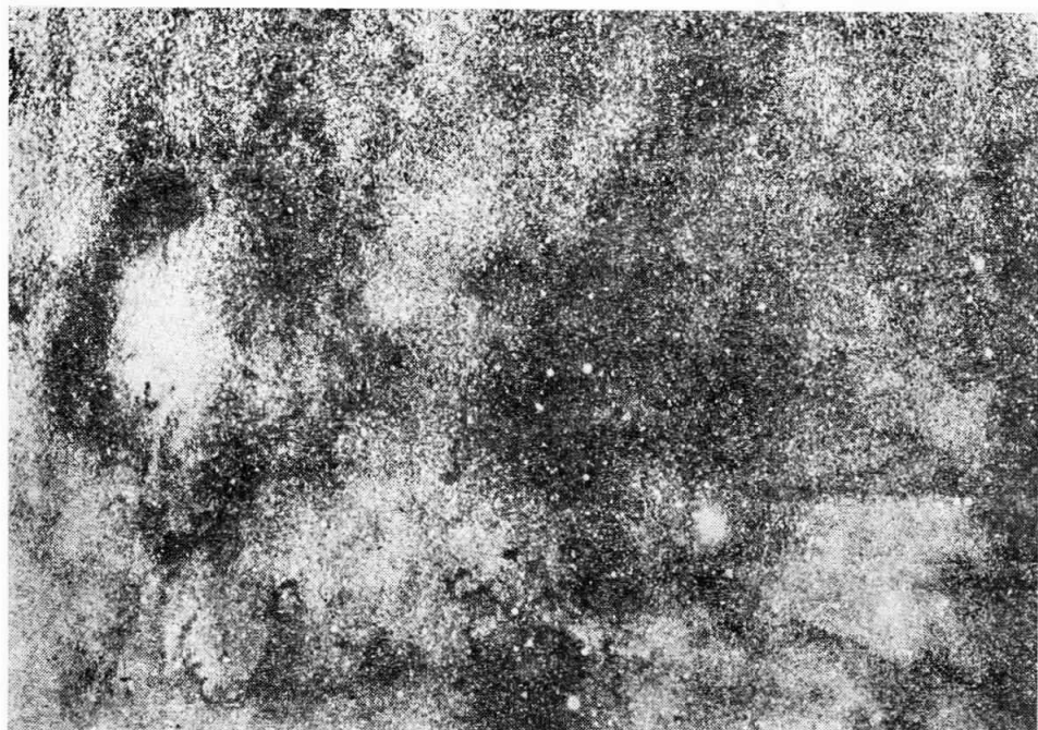
Εἰκ. 3. Τμήμα τοῦ Γαλαξίου εἰς τὸν Ὀφιοῦχον, ὅπου διακρίνεται καὶ σκοτεινὸν νέφος.
