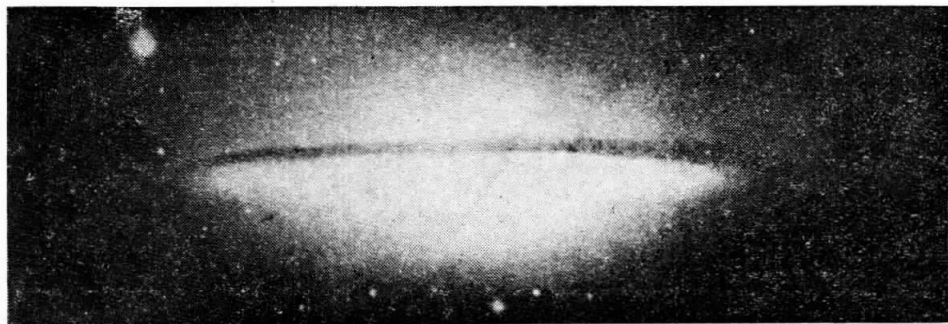
Εἰκ. 2. Σπειροειδῆς Γαλαξίας τῆς Παρθένου, ὁρώμενος πλαγίως. Λόγω τῆς μεγάλης ἀποστάσεως—22.000.000 ε. φ.—δὲν διακρίνονται εὐκόλως οἱ αστέρες του. Εἰς τὸ μέσον βλέπομεν σκοτεινὸν νέφος τὸ ὁποῖον τὸν περιβάλλει και φαίνεται ὡς ἕαν τὸν διαιρεῖ εἰς δύο μέρη.
